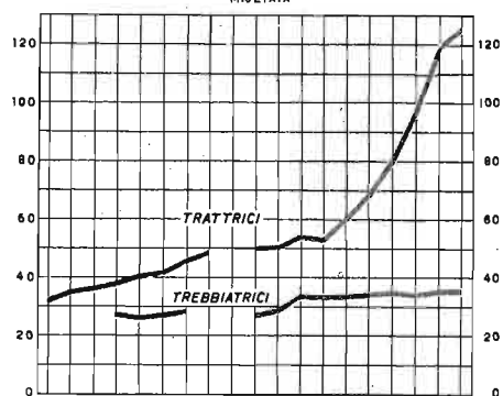
TRATTRICI, TREBBIATRICI E CONSUMO DI CARBURANTI PER USO AGRICOLO NEGLI ANNI DAL 1936 AL 1954
